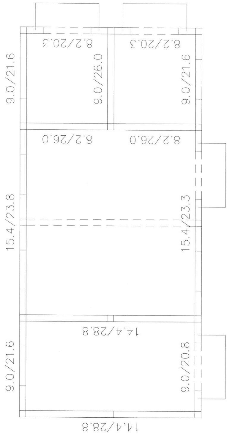
附图 2-3 一层墙体高厚比
