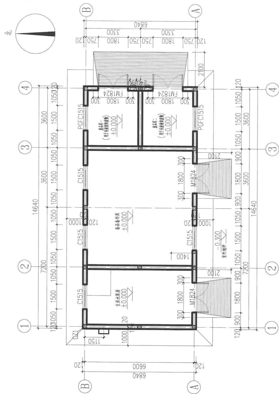
附图 1-1 一层平面布置图
